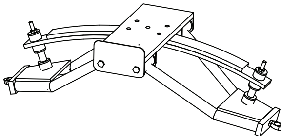
A-Arm Assembly
